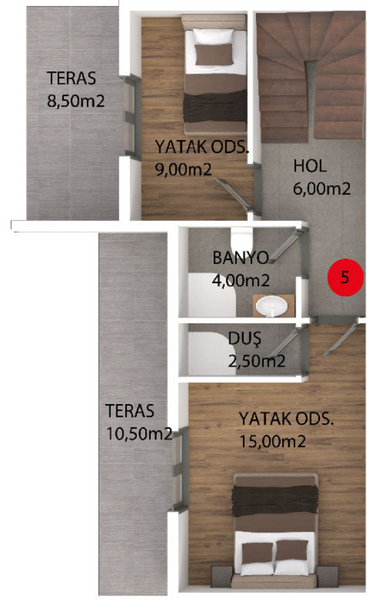
ÜST KAT
